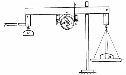
Schéma du dispositif d'essais de G.A.Hirn (1854)
